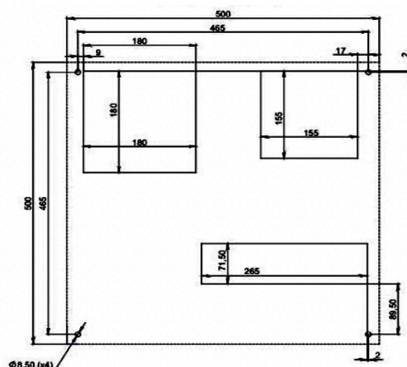
Монтажный вырез для установки кондиционера 0.5-0.8 кВт серия "В" (вид снаружи)
