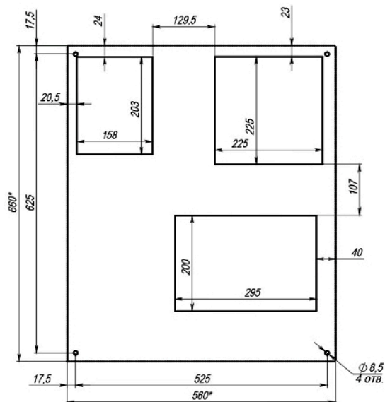
Монтажный вырез с внешней стороны (со стороны кондиционера) для кондиционера 1.0-1.5 кВт серии "В"
