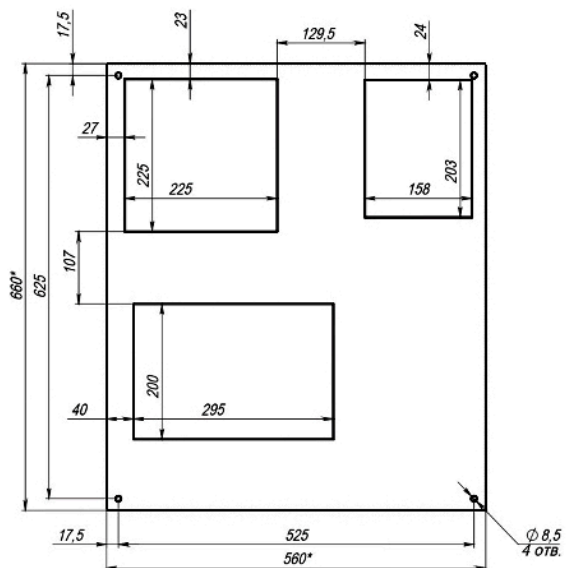
Монтажный вырез с внутренней стороны (со стороны шкафа) для кондиционера 1.0-1.5 кВт серии "В"
