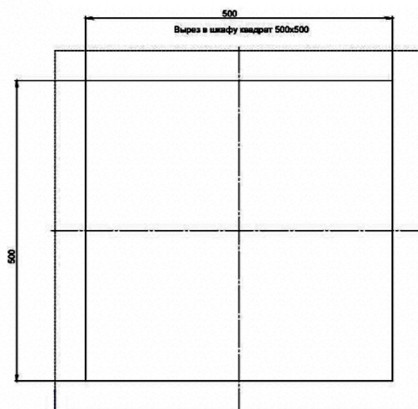
Монтажный вырез для установки кондиционера 0.5-0.8 кВт серия "В" (монтаж под уголки)
