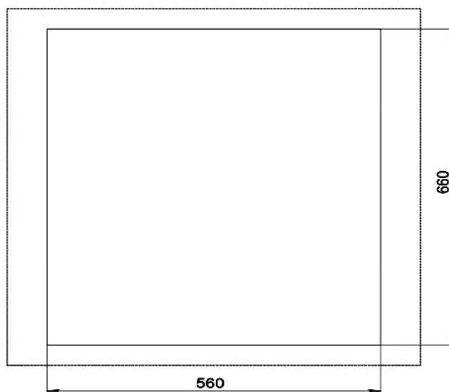
Монтажный вырез под кожух для установки кондиционера 1.0-1.5 кВт серии "В" Прямоугольный вырез в шкафу 660x560мм
