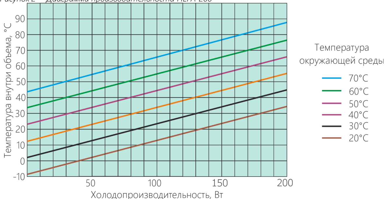
Рисунок 2 - Диаграмма производительности НЕГА-200
