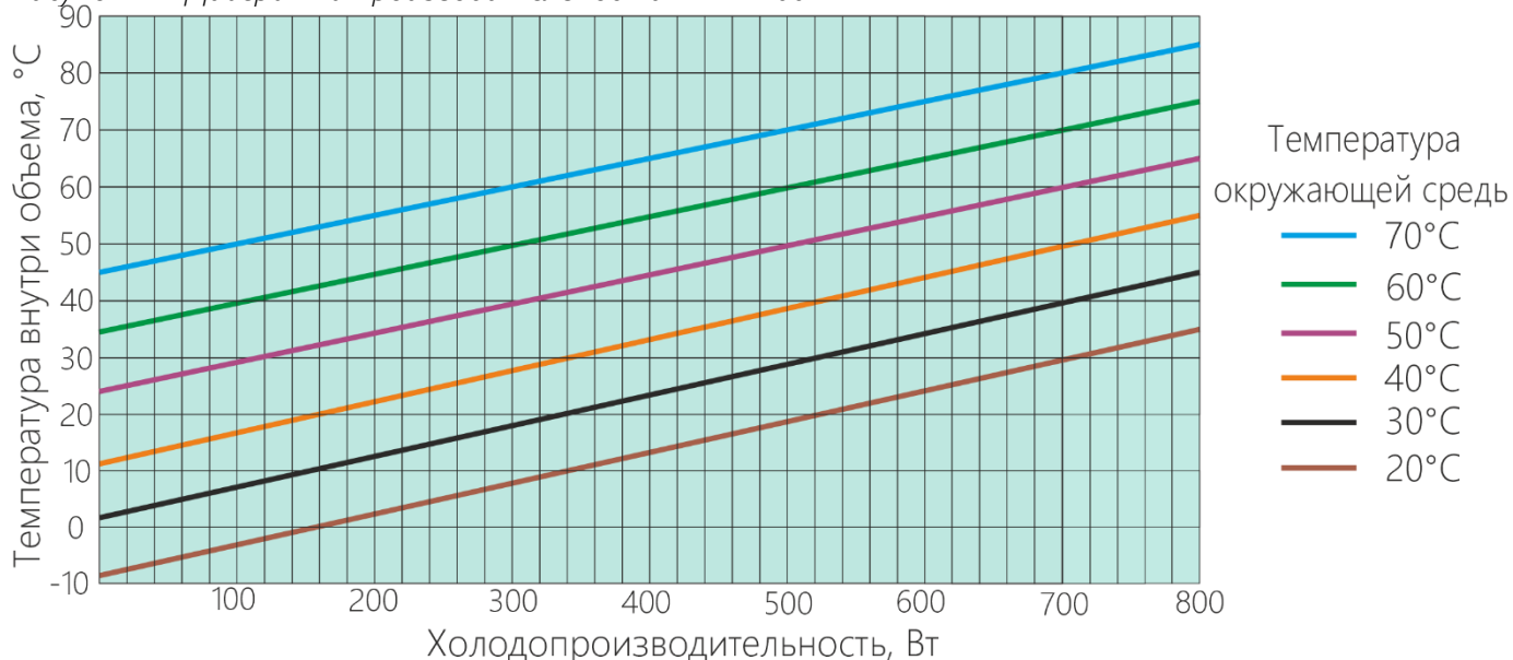
Рисунок 2 - Диаграмма производительности НЕГА-400
