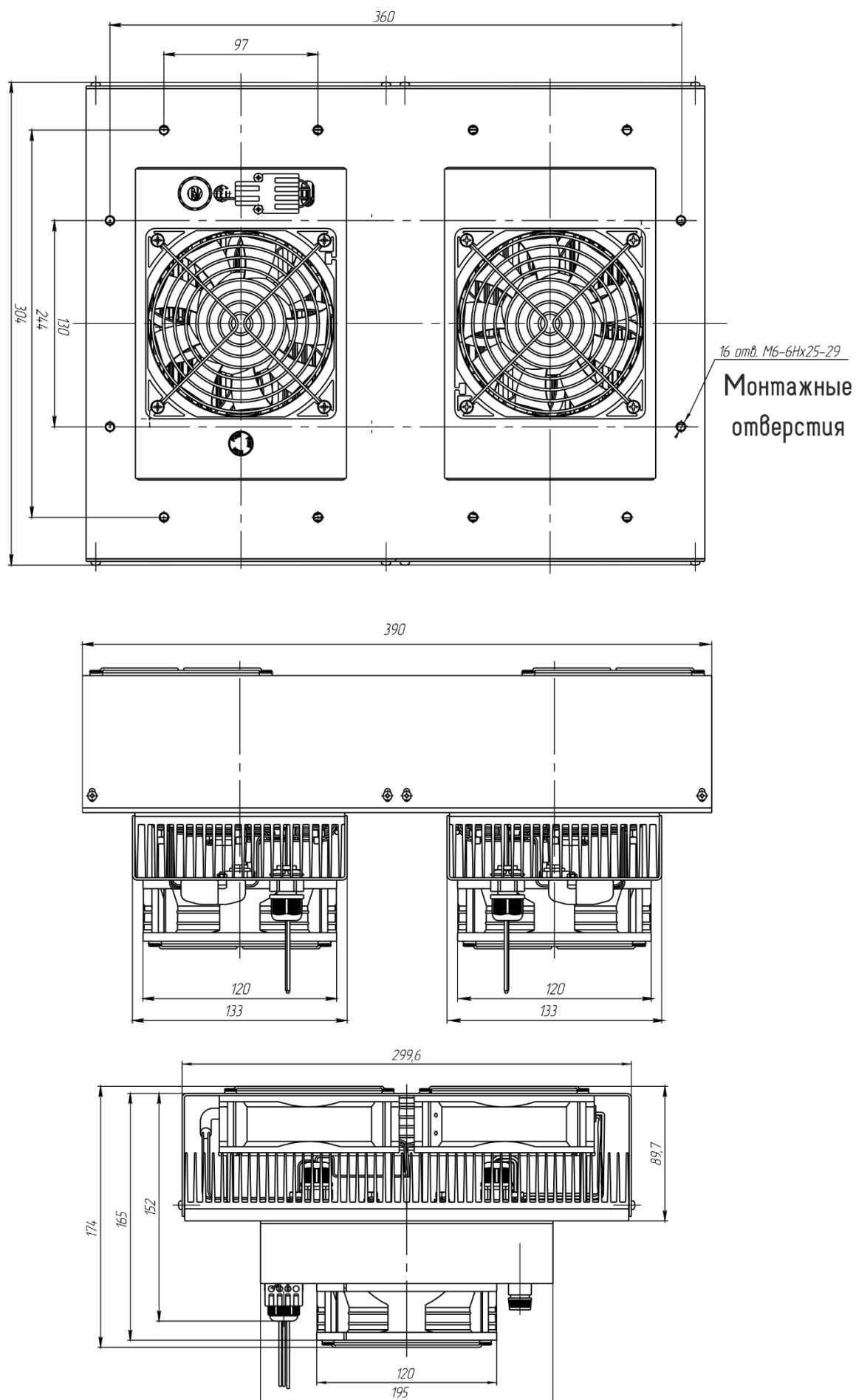
Рисунок 1 – Габаритные и другие размеры изделия
