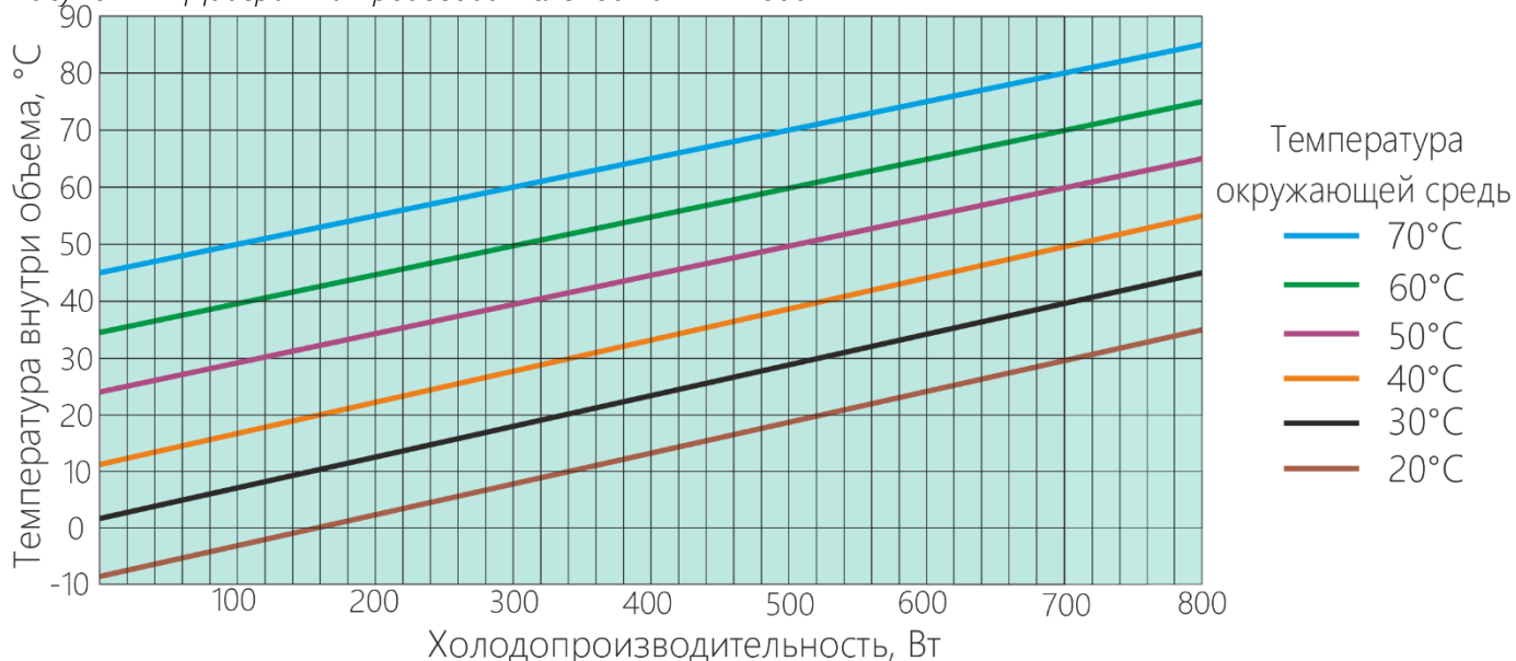
Рисунок 2 - Диаграмма производительности НЕГА-800
