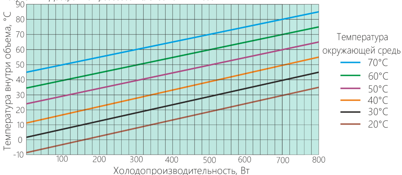
Рисунок 2 - Диаграмма производительности НЕГА-600
