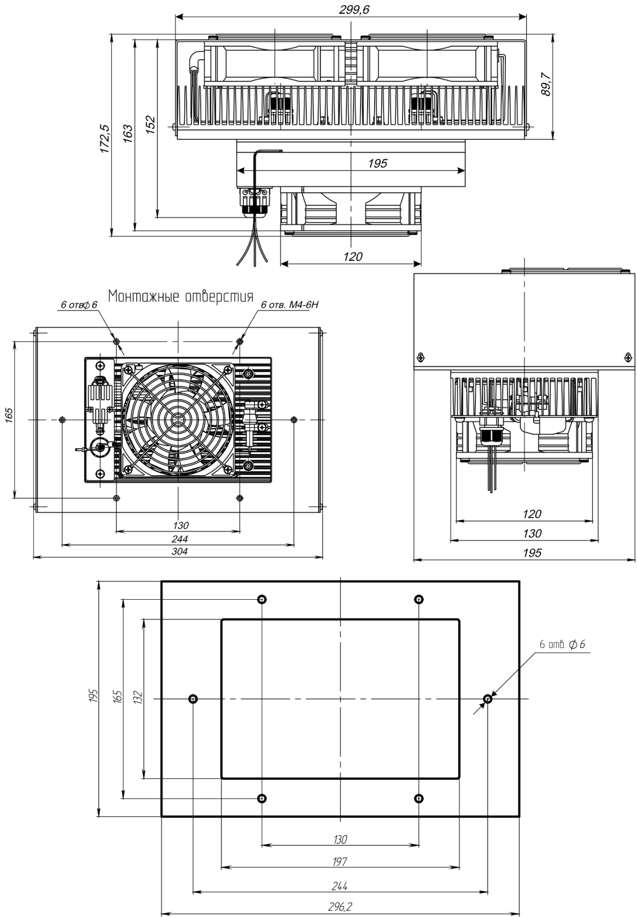
Рисунок 1 - Общий вид изделия
