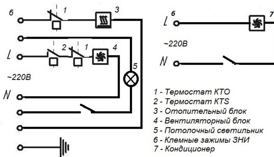
Рис. 5. Схема электрическая
