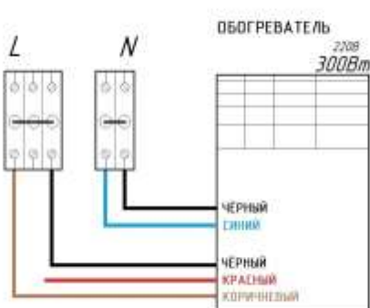
Рисунок: Структурная схема климатической системы
