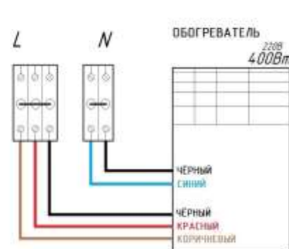
Рисунок: Структурная схема климатической системы
