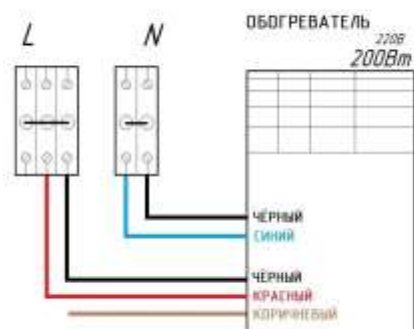
Схема подключения 1.
