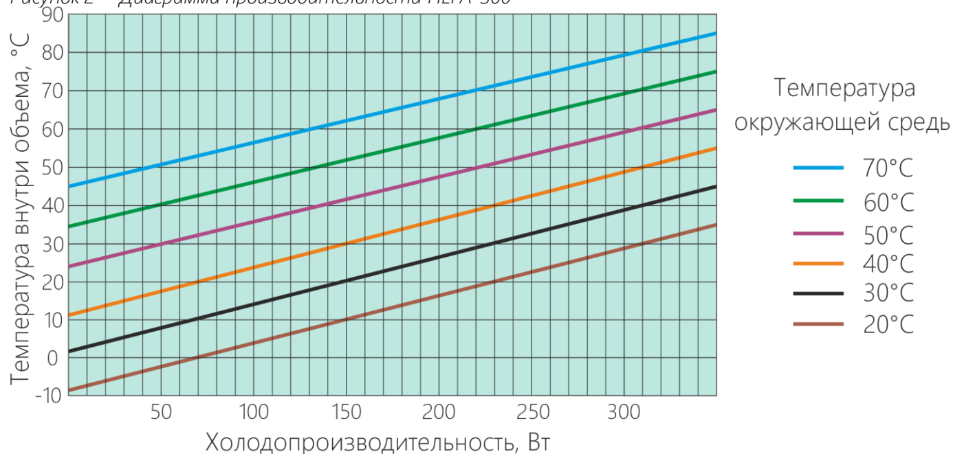
Рисунок 2 - Диаграмма производительности НЕГА-300
