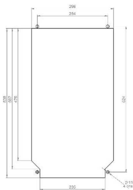
Монтажный вырез полуутопленный монтаж
