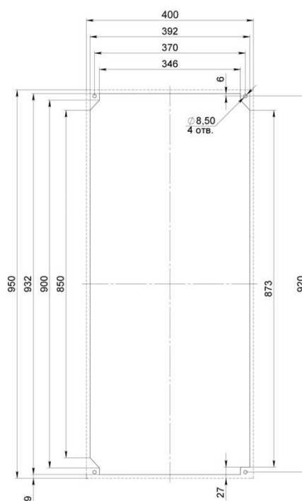
Монтажный вырез утепленный монтаж
