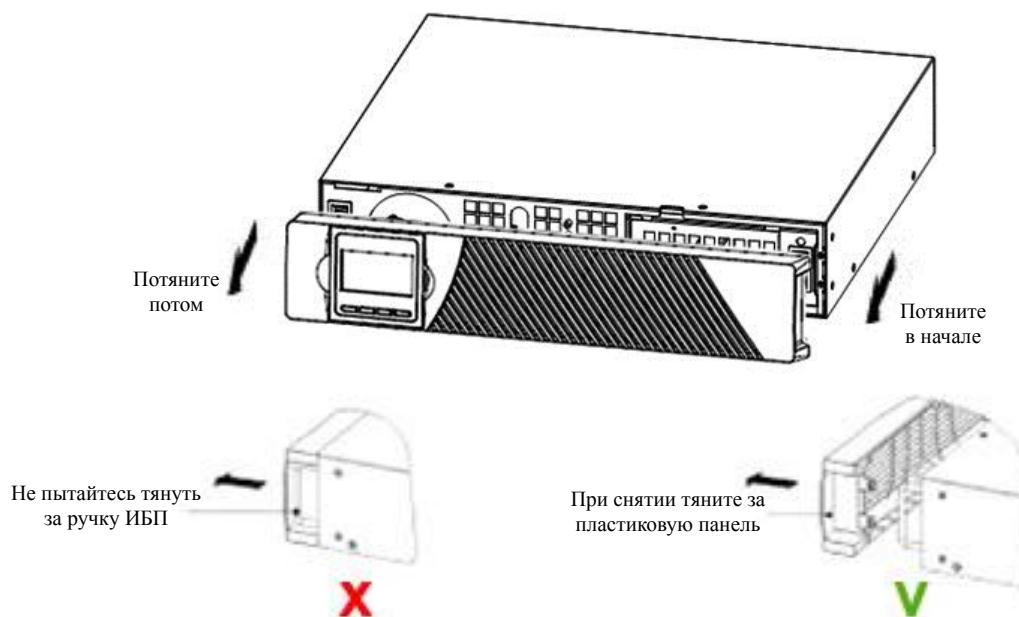
Рисунок 8 Снятие передней панели
