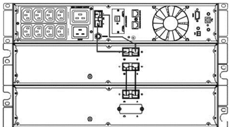
Подключение на задней панели (опционально, модели ИБП без встроенных аккумуляторов)
