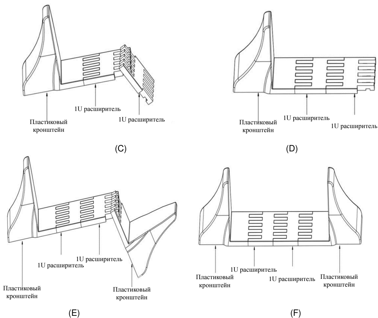
Рисунок 12 Расширение базы подставки
