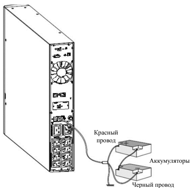
Рисунок 16 Подключение внешних батарей к ИБП с увеличенным временем работы
