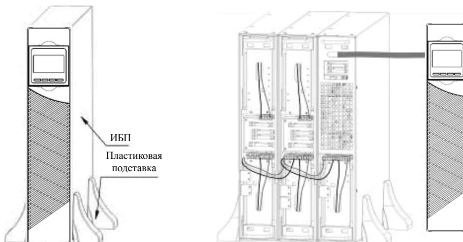
Рисунок 14 Напольная установка ИБП и батарейных блоков
