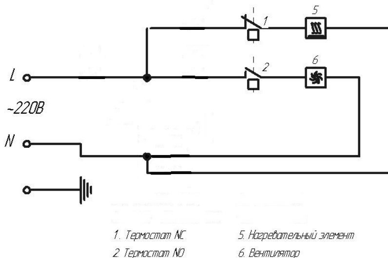
Рис. 5. Схема электрическая
