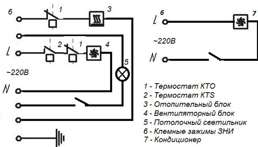
Рис. 5. Схема электрическая
